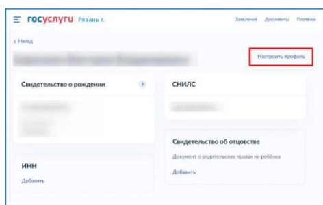
Рисунок 17. Настройка профиля
